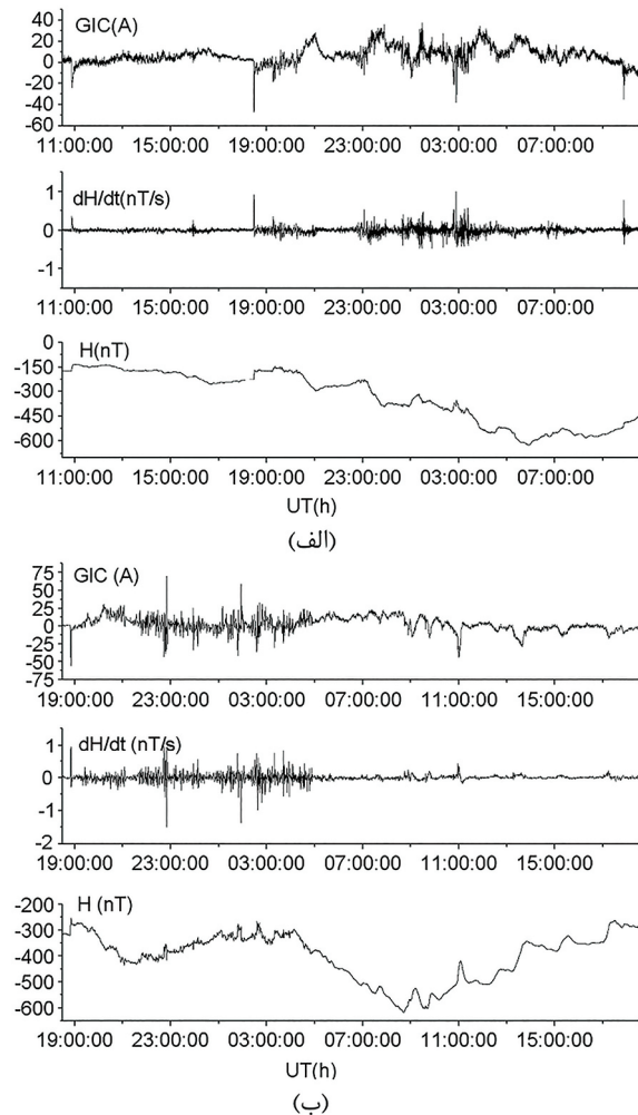
شکل ۱: داده‌های GIC، مؤلفه افقی و تغییرات زمانی مؤلفه افقی میدان مغناطیسی ثبت شده در نیروگاه هسته‌ای لینک آئو به همراه مؤلفه افقی میدان ژئومغناطیسی از رصدخانه ژائوکینگ در (الف) ۸-۷ و (ب) ۹-۱۰ نوامبر ۲۰۰۴ [۱۹].
