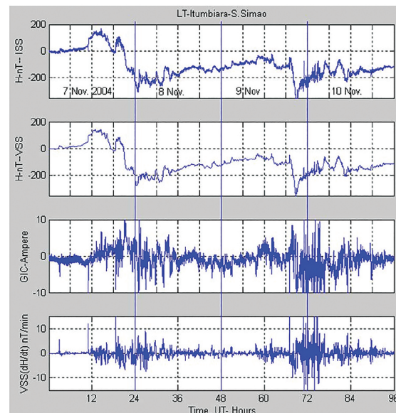
شکل ۴: تغییرات مؤلفه افقی میدان مغناطیسی H، تغییرات GIC محاسبه شده در طوفان مغناطیسی در بازه زمانی ۷ تا ۱۰ نوامبر ۲۰۰۴ در زیر خط انتقال ایتومبیرا-سیمائو سائو و در ایستگاه مرجع و dH/dt در ایستگاه مرجع است [۳].
