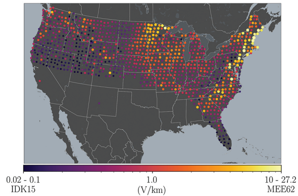
شکل ۹: پیش‌بینی رویداد طوفان ژئومغناطیسی شدید یکبار در قرن از میدان ژئوالکتریک اندازه‌گیری شده در سایت‌های مگنوتلوریک در ایالات متحده آمریکا. مناطق با خطر بالا و کم در سراسر کشور وجود دارند که پیچیدگی ژئوالکتریک ایالات متحده را نشان می‌دهد [۲۱].
