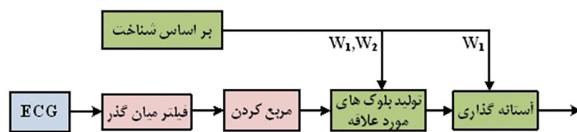
شکل ۱۷: دیاگرام بلوکی الگوریتم تشخیص QRS بر اساس شناخت [۲۵]
