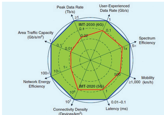
شکل ۲: مقایسه مشخصات فنی ارتباطات در نسل پنجم و ششم
