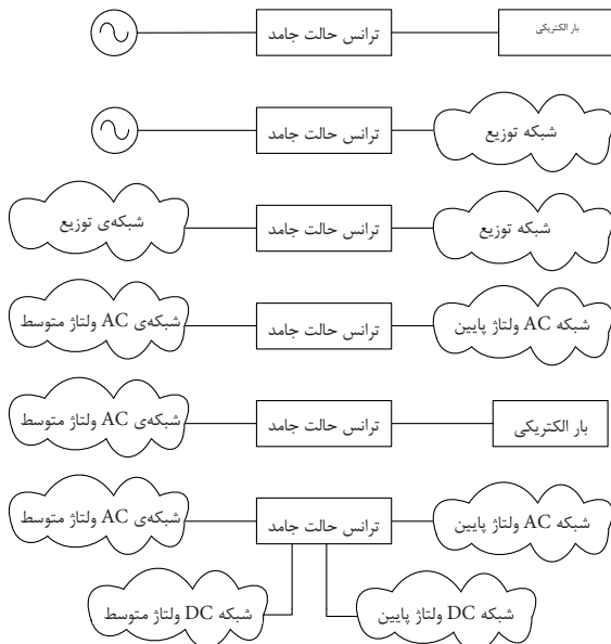
شکل ۶: کاربردهای SST در شبکه قدرت
