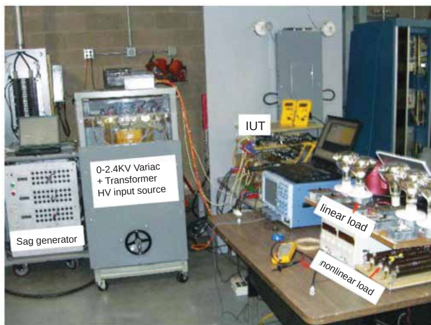
شکل ۱۰: نمونه آزمایشگاهی IUT ساخته شده توسط EPRI [۱۸]
