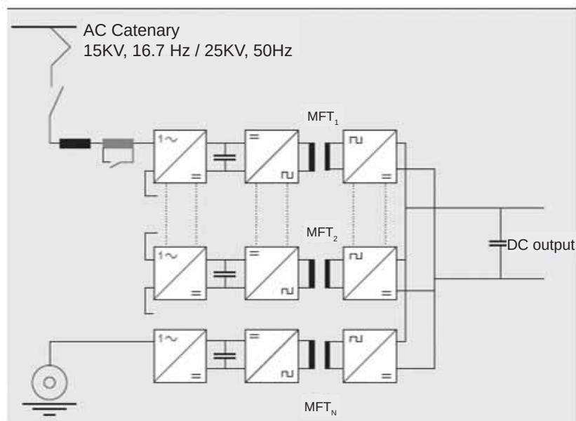
شکل ۱۱- ساختار بلوکی ترانس پیشنهادی ABB [۱۵]
