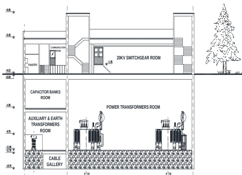
شکل ۳: مقطع طولی (B-B) پست 132/20kV میدان شهدا مشهد
