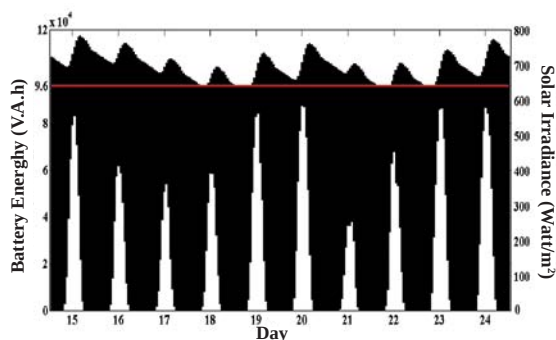
شکل ۹: منحنی انرژی ذخیره شده در باتری (سطح سفید رنگ) و میزان تابش نور خورشید (سطح سفید رنگ) یا در نظر گرفتن ضریب اصلاحی پل
