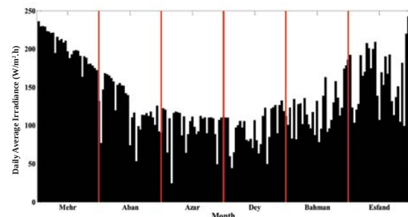
شکل ۷: میانگین تابش روزانه در ۶ ماهه دوم سال
