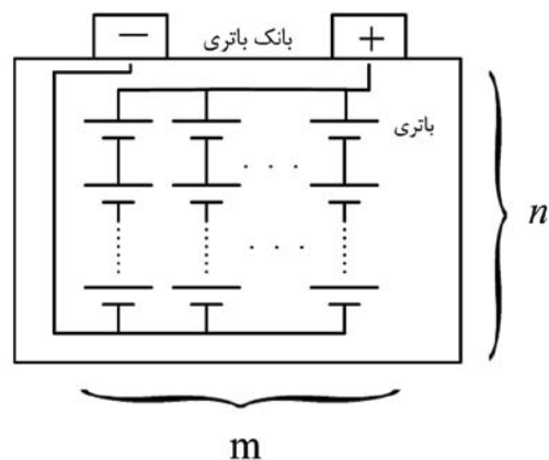
شکل ۵: شکل ساده شده بانک باتری متشکل از باتری های سری و موازی
