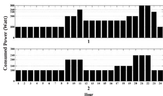
شکل ۵: الگوی بار مصرفی ۵ خانوار روستایی: (۱) ۶ ماهه اول (۲) ۶ ماهه دوم
