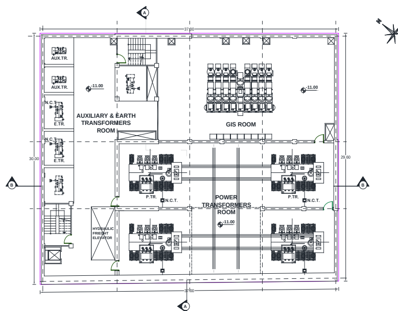
شکل ۱: پلان طبقه ۲- پست 132/20kV میدان شهدا مشهد (۲ ترانس قدرت و ۲ ترانس زمین به صورت توسعه در نظر گرفته شده‌اند)
