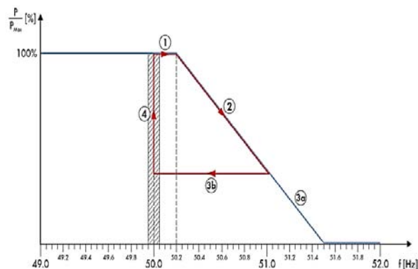
شکل ۸: تغییرات توان نسبت به فرکانس در اینورتر نیروگاه
