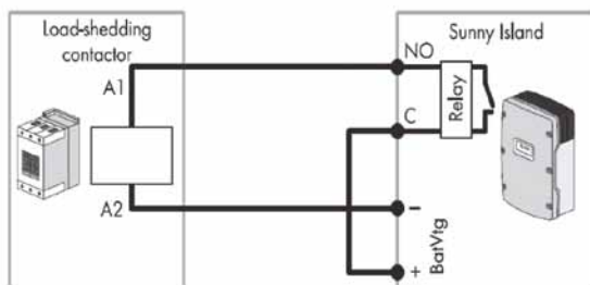
شکل ۷: حذف بار در ریز شبکه
