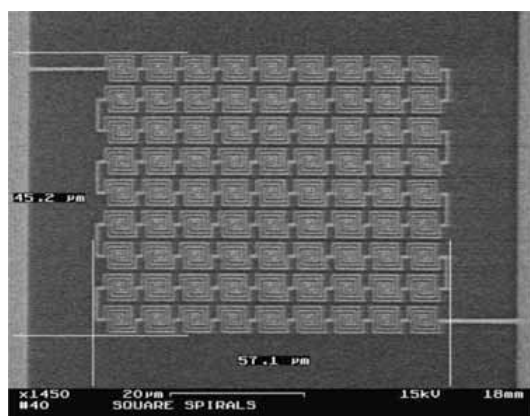
شکل ۳: (الف) نانوانتن مارپیچی متصل به یکسوساز و (ب) آرایه‌ی دو بعدی نانوانتن‌های مارپیچی جهت جمع‌آوری انرژی خورشیدی [۵]
