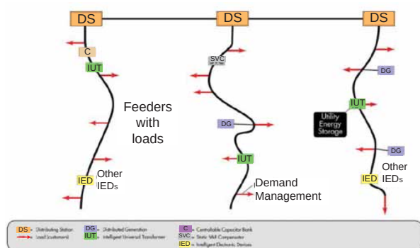
شکل ۹: نمایش مفهومی شبکه توزیع برق هوشمند [۱۸]
