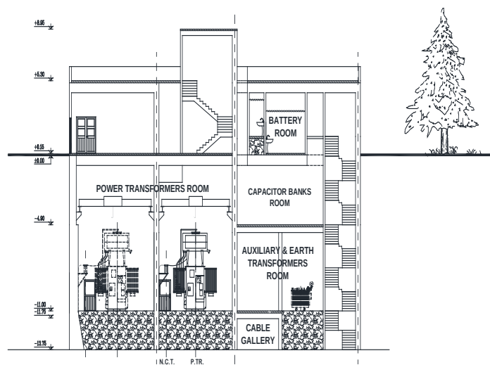
شکل ۲: مقطع عرضی (A-A) پست 132/20kV میدان شهدا مشهد
