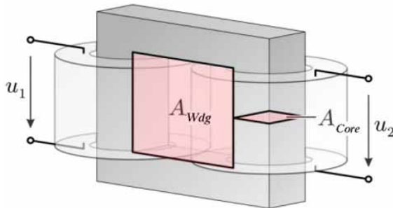
شکل ۳: ساختار کلی هسته ترانسفورماتور
