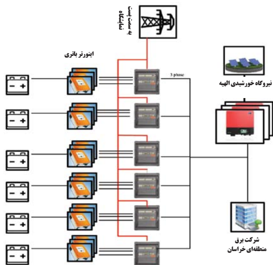
شکل ۶: ساختار ریز شبکه
