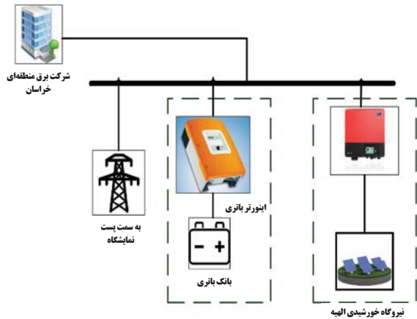
شکل ۳: ساختار کلی برای اضافه کردن سیستم باتری
