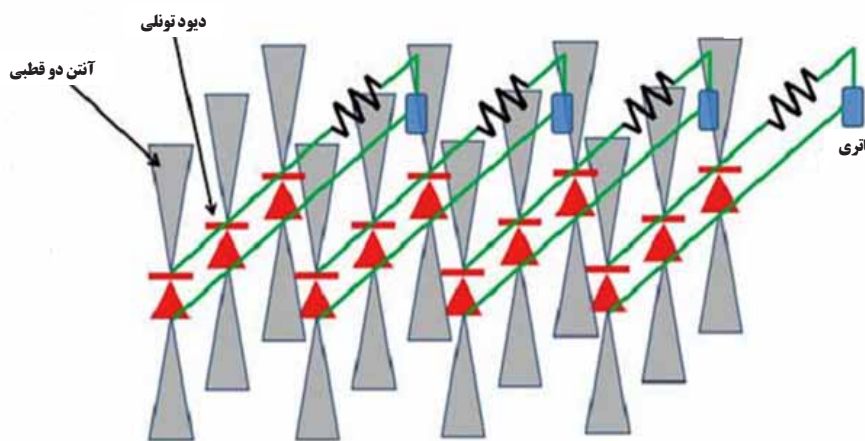
شکل ۱: طرح شماتیک یک مجموعه رکتن خورشیدی متشکل از نانوآنتن های دوقطبی
