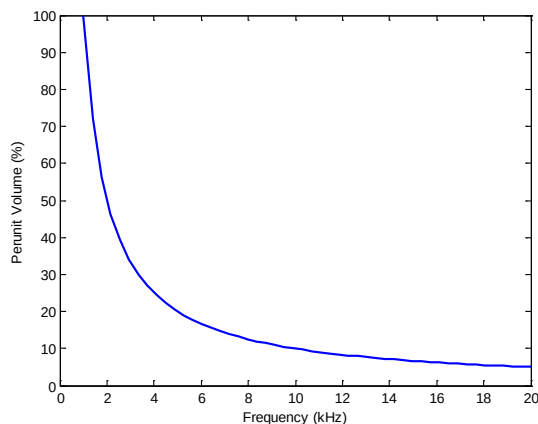
شکل ۴: حجم هسته در فرکانس‌های کاری مختلف نسبت به فرکانس ۱ kHz
