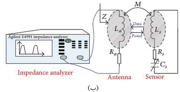
شکل ۱۳: (الف) مدار و (ب) تصویر سنسور فشار با استفاده از خازن بین انگشتی [۳۰]
