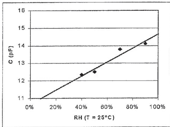
شکل ۵: (الف) سنسور رطوبت-سنج با استفاده از لایه جاذب رطوبت [۱۳، ۱۲] و (ب) ظرفیت خازن برحسب رطوبت نسبی موجود در دمای ۲۵°C [۱۵]
