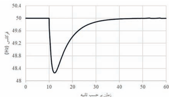
شکل ۹: فرکانس شبکه توزیع در حالت جزیره‌ای برای سناریوی اول
