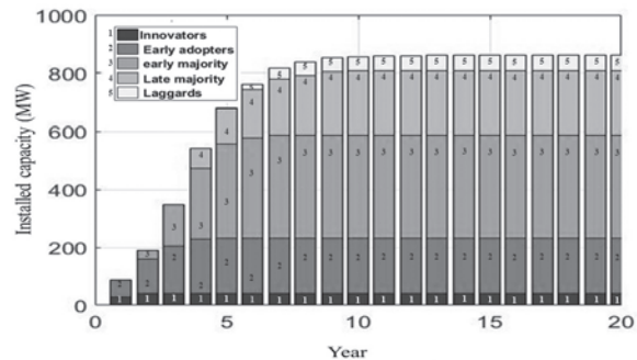
شکل ۸: نتایج شبیه سازی نفوذ فتوولتائیک حالت پایه
