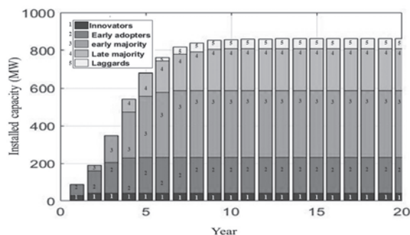
شکل ۸: نتایج شبیه سازی نفوذ فتوولتایک حالت پایه
