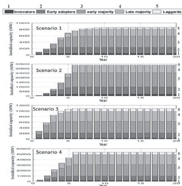
شکل ۷: نتایج شبیه سازی نفوذ نیروگاه های فتوولتایک در سناریوهای طرح شده سیاست تلفیقی
